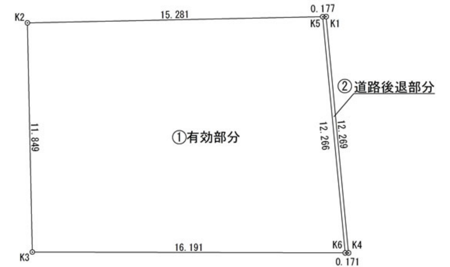
求積図 縮尺 1/200
